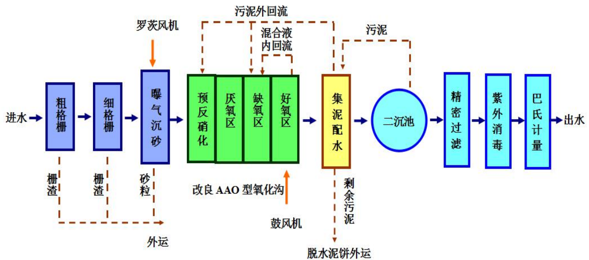
图 5-1 三灶厂环保设施运行流程图
